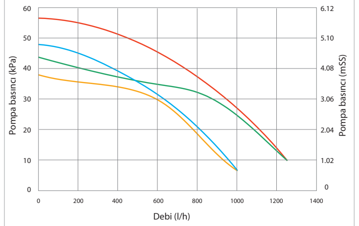
Debi (akış oranı) ve Basınç Grafiği
